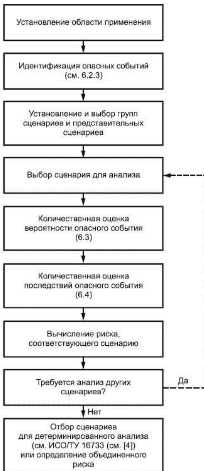
Рисунок 2. Схема оценки пожарного риска
